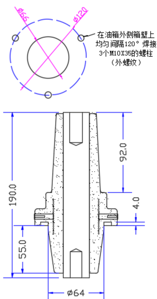
油箱开孔尺寸
